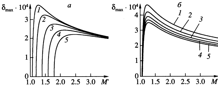
Фиг. 6. Графики функций \delta_{\max}(M) при \mu = 1.2 \cdot 10^{-4} ; а: D = 23.9 , M_w = 0, 0.2, 0.4, 0.6, 0.8 (кривые 1–5); б: M_w = 0 , D = 10, 15, 20, 25, 30 (кривые 1–5)
